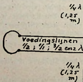
Vertikale stroomgevoede dipool voor 5 meter.
