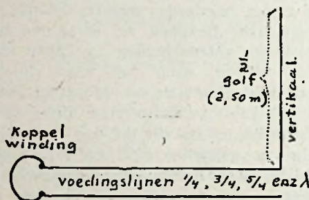
Vertikale „Zeppelin”-antenne voor 5 meter.
